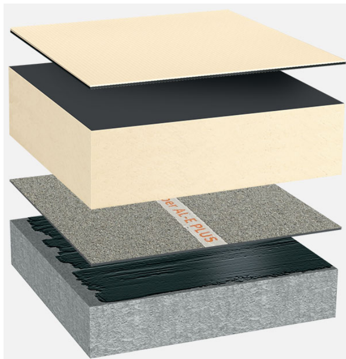
Soluzioni sistema: BG_PIR-FA_T_02
