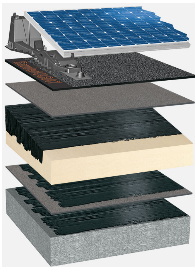
Soluzioni sistema: BP_PIR-KG_K_01_PVFD
