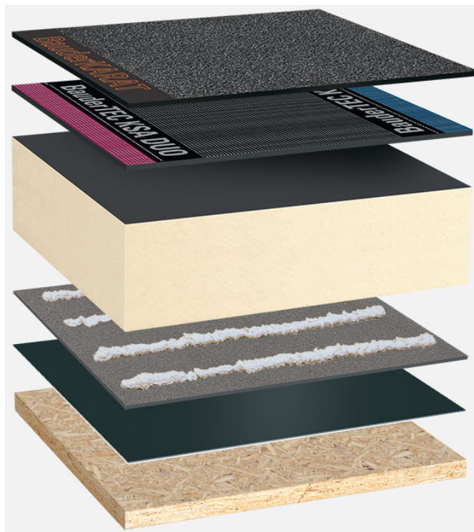
Soluzioni sistema: HG_PIR-FA_K_02
