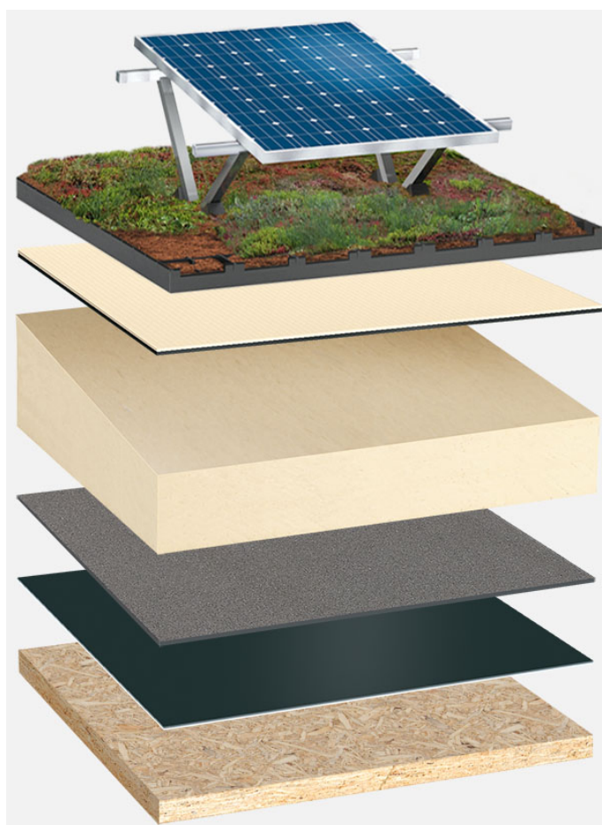
Soluzioni sistema: HP_PIR-TG_T_01_PVGD
