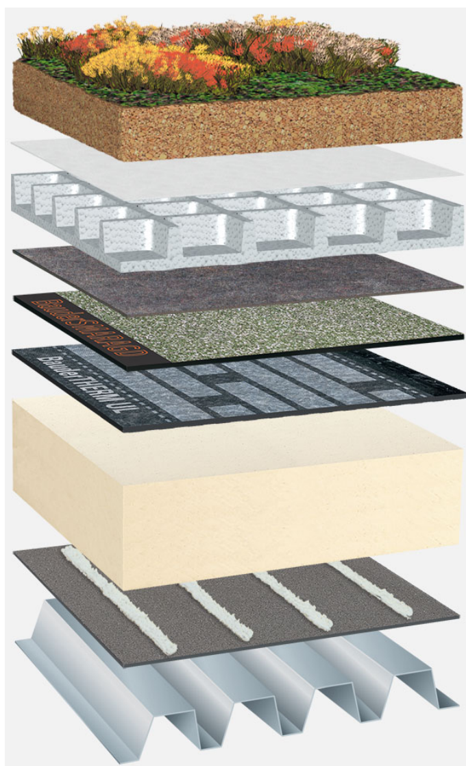
Soluzioni sistema: TG_PIR-MF_S_01_G75
