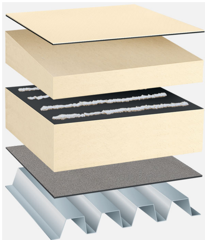
Soluzioni sistema: TP_PIR-FA_PIR-TG_T_01
